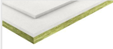
fermacell Estrich-Element 2 E 32 (2 E 34) 2 x 10 mm fermacell Gipsfaser-Platte + 10 mm Mineralwolle
